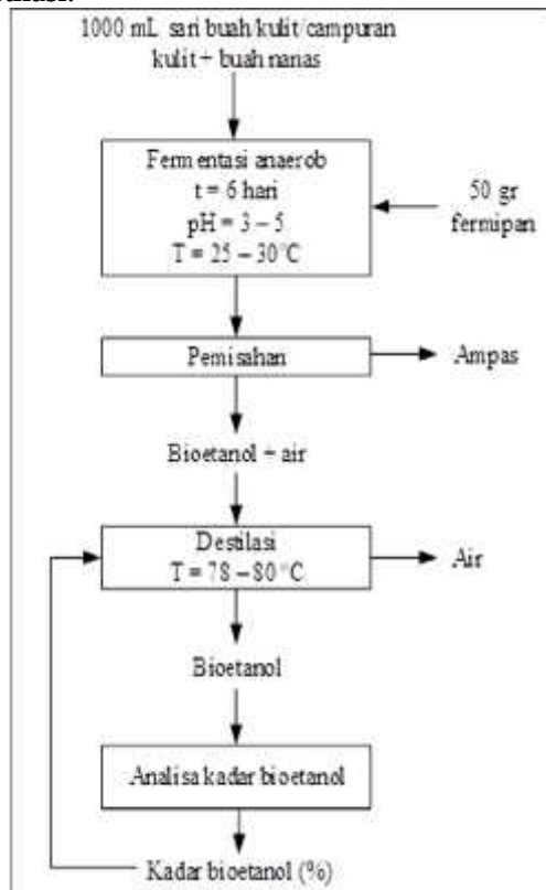
Gambar 2. Blok Diagram Proses Fermentasi dan Operasi Destilasi
