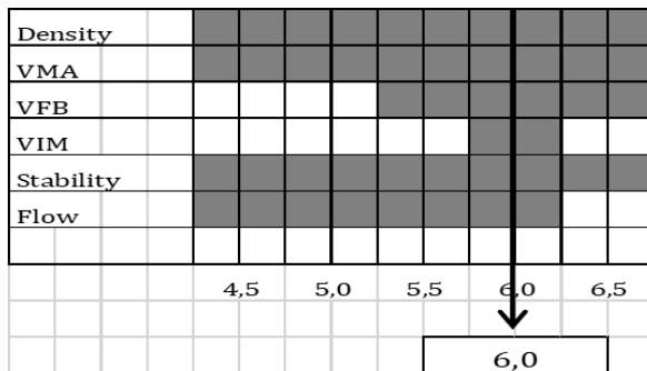
Gambar 1. Penentuan Kadar Aspal Optimum (KAO)
